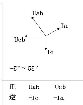
A、C相电流相间接错并接反
