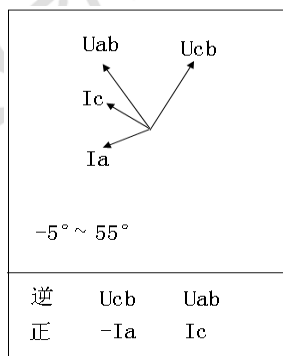
A、C相电压接反
