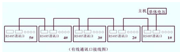
图 2.4.4.4 有线通讯口接口图
