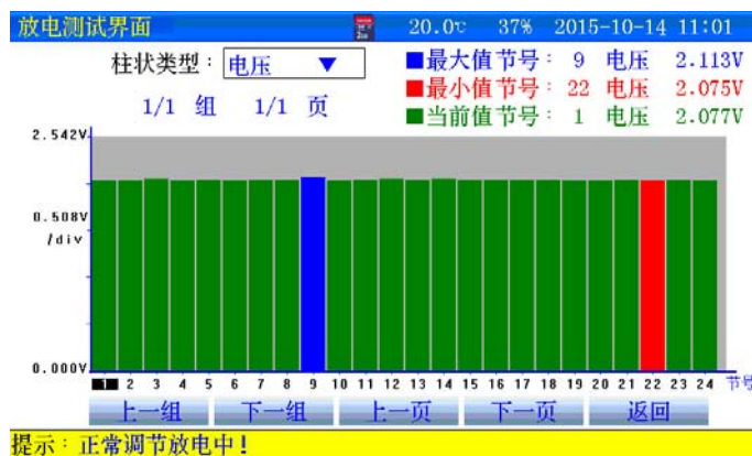
图 3.2.4-1 单体电压柱状图
