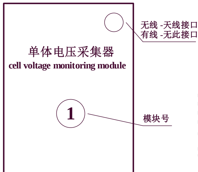
图 2.4.3 单体模块正图
