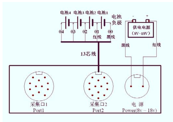
图 2.4.4-2 4 节 12V 电池与 1 个单体模块连接图
