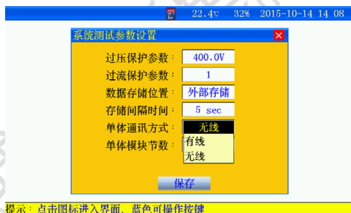
图 3.13 主机与单体模块通讯方式设置界面
