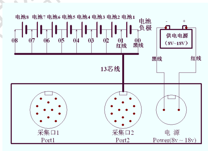
图 2.4.4-1 8 节 6V 电池与 1 个单体模块连接图
