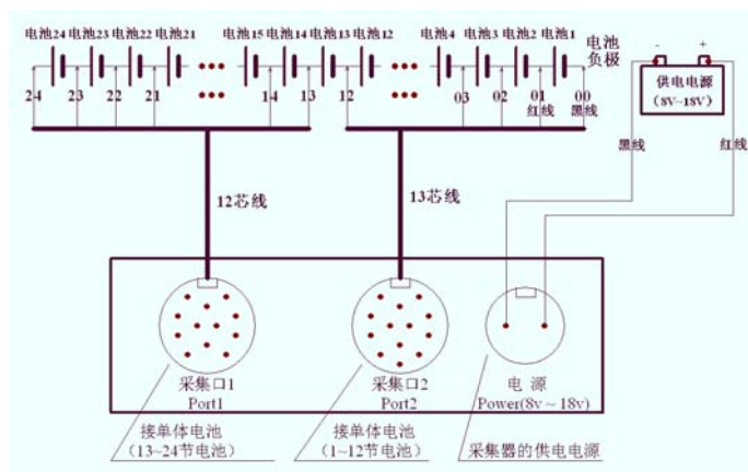
图 2.4.4 24 节 2V 电池与 1 个单体模块连接图
