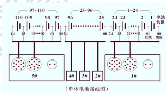
图 2.4.4-3 多个单体模块与电池连接图
