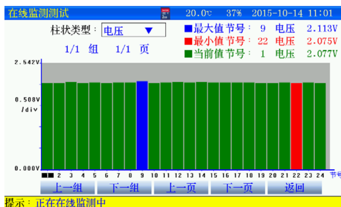
图 3.1.4-1 单体电压柱状图
