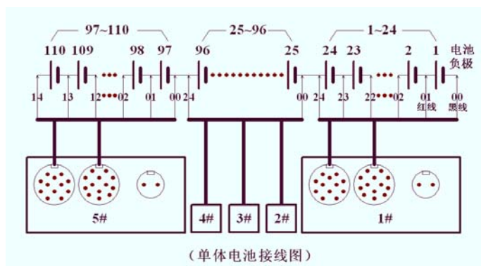
图 2.4.4-3 多个单体模块与电池连接图
