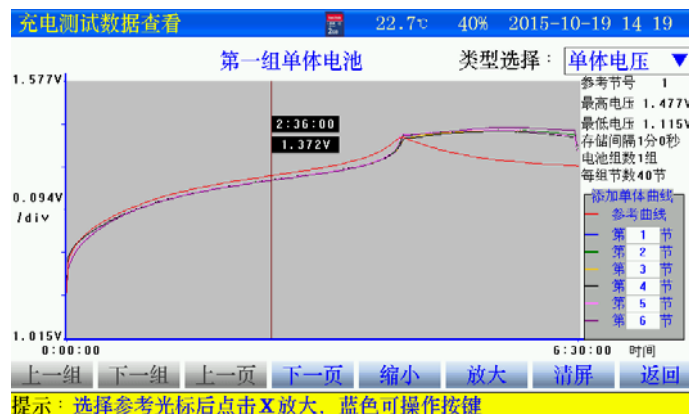
图 3.4.4-1 单体电压曲线界面
