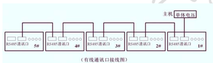
图 2.4.4-4 有线通讯口接线图
