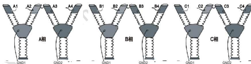
十二断口信号线的连接
