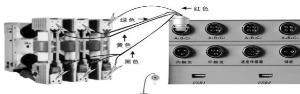
断口接线图（六断口）
