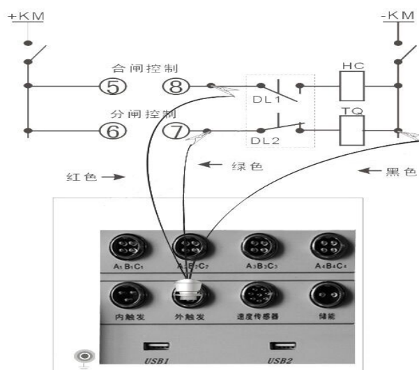
高压开关控制屏外触发控制接线示意图
