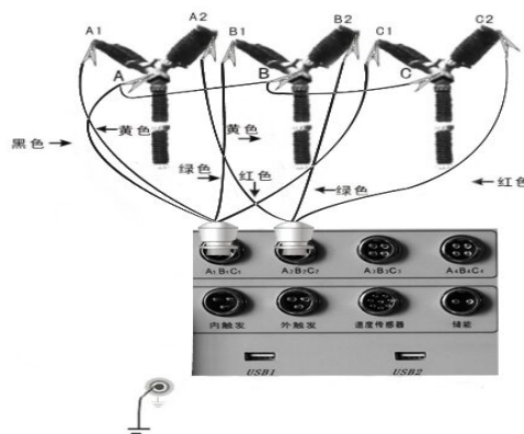
断口接线图（六断口）
