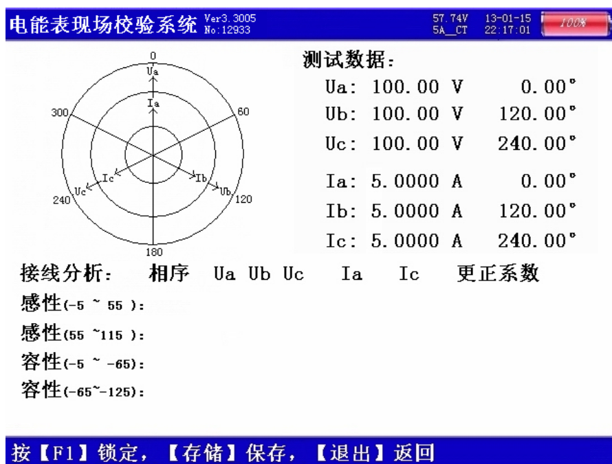
图九、矢量分析屏—三相四线
