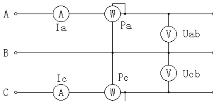
图二十、三相三线计量原理图
