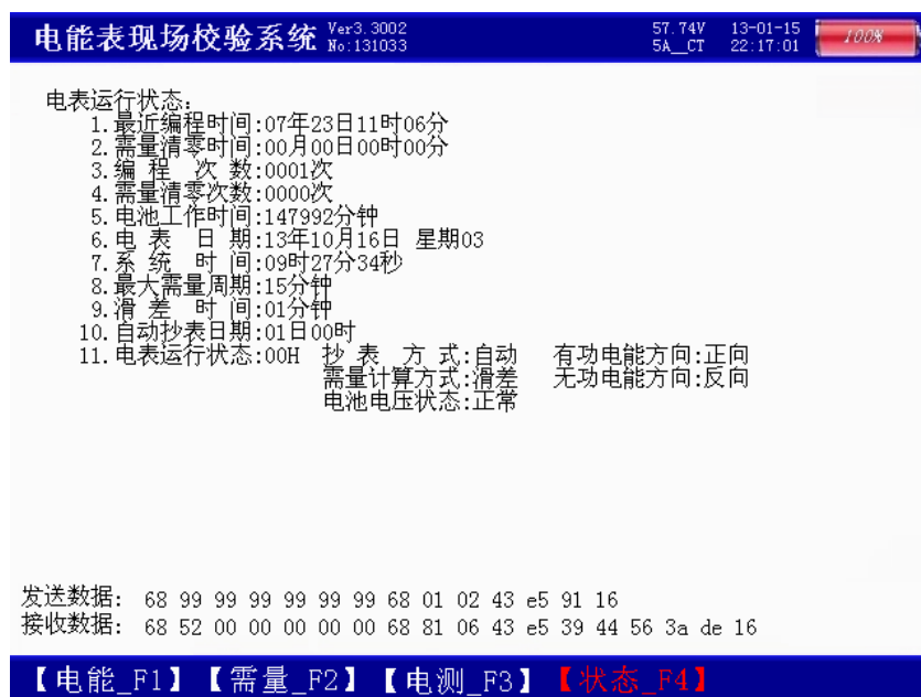
图十五、测试_485 状态
