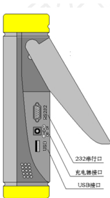
图二、仪器侧面图
