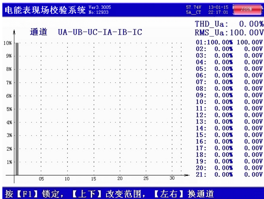
图十七、频谱分析屏
