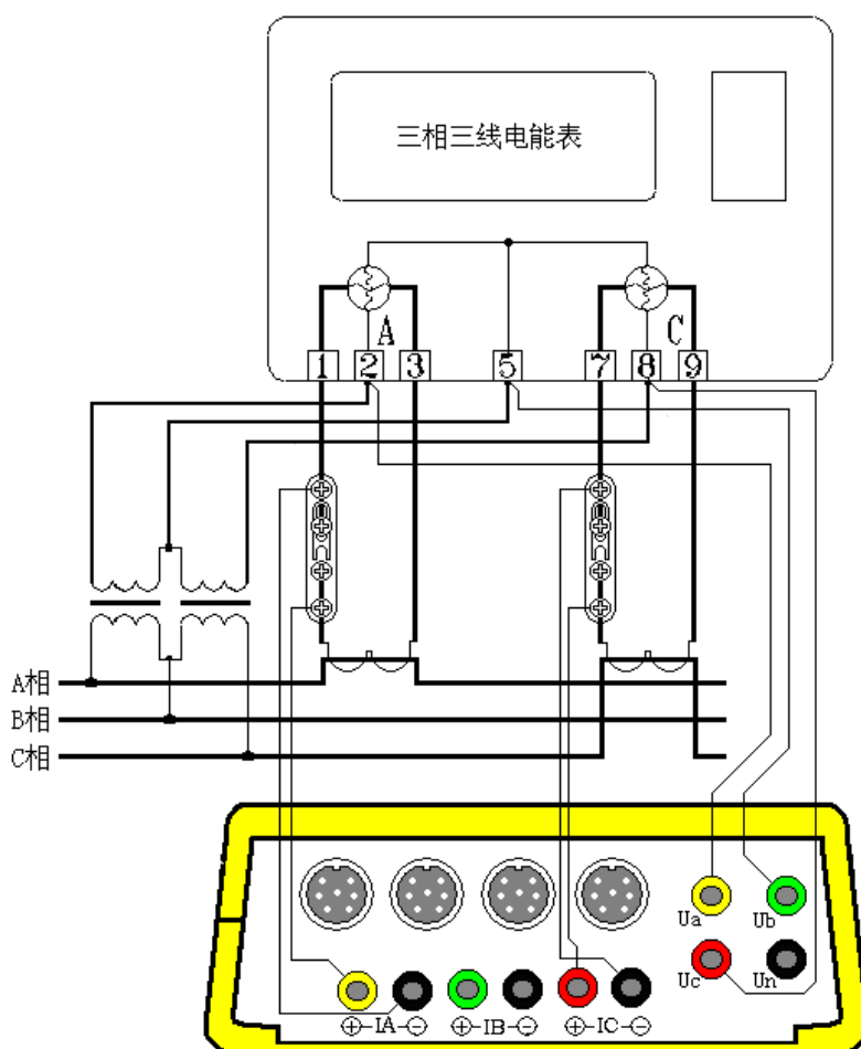
三相三线高压表计经内部CT接线
