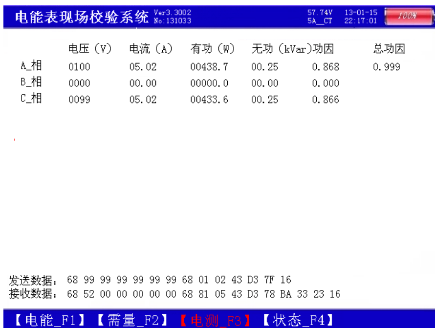
图十四、测试_485 电测
