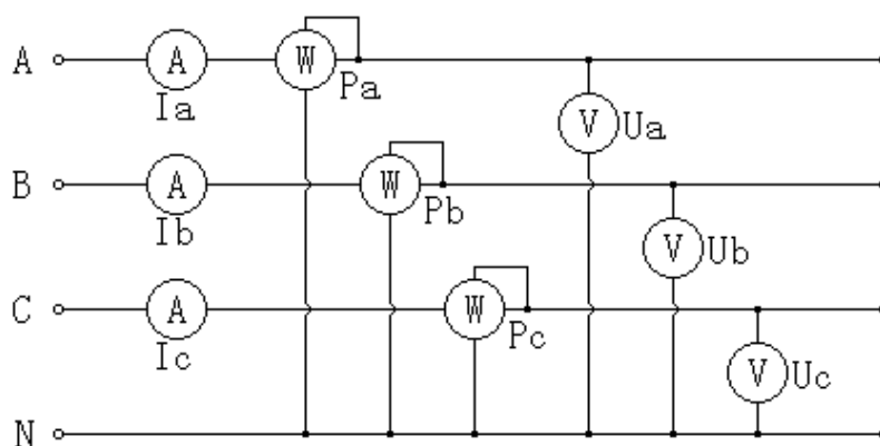
图二十一、三相四线计量原理图
