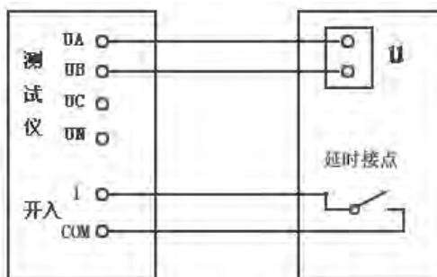
时间继电器接线
