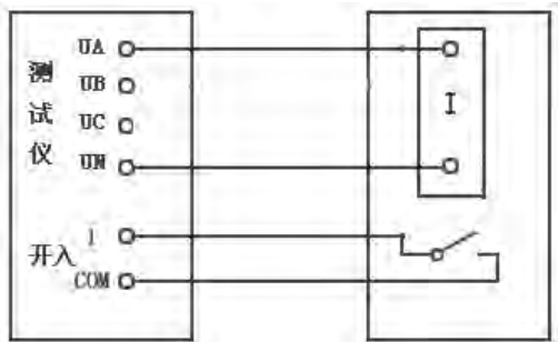
信号继电器接线
